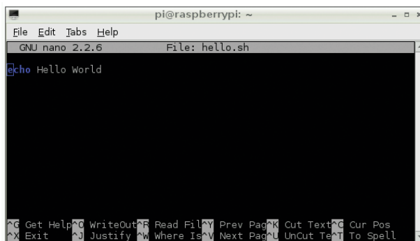
Figure 4.4. Nano.
